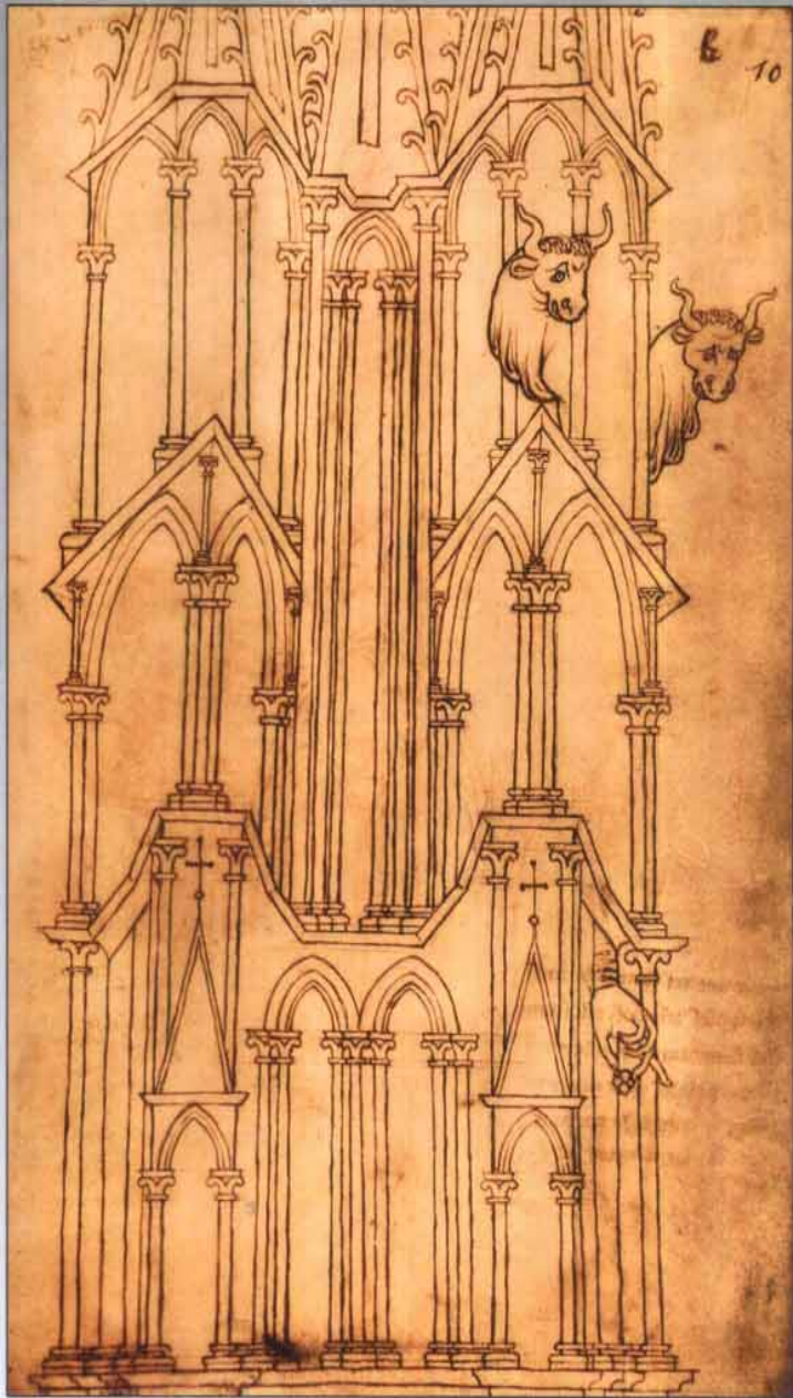
这幅拉翁大教堂塔楼的草图，绘制了两尊公牛的雕像，有可能是在建筑中用来使人联想到野兽，但是右边绘制的那只手却是奥诺古尔本人的奇想。
